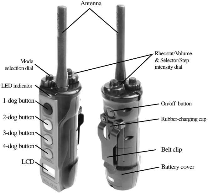
EDGE Transmitter
